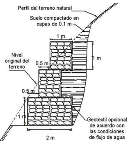
Figura 2-45. Muro en gaviones de piedra
