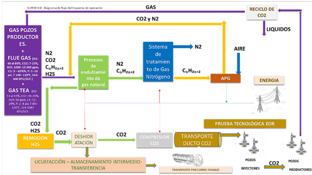
Figura 2-86 Diagrama de Flujo del Esquema de Operación: Captura e inyección de CO2
