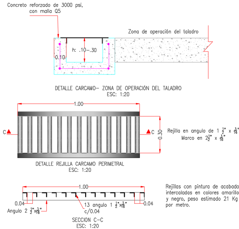
Figura 2-64 Cárcamo perimetral
