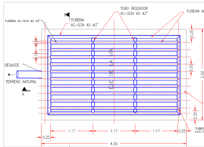
Figura 2-48 Quiebrapatras
