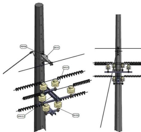
Figura 2.144 Estructuras de suspensión con ángulo de 35 grados
