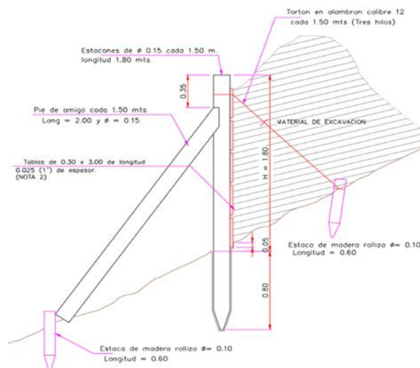
Figura 2-47. Trinchos laterales tipo
