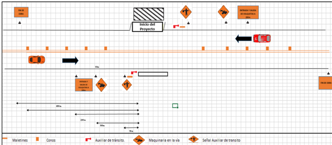
Figura 2-57 Esquema Típico de Señalización para Mantenimiento de Vía
