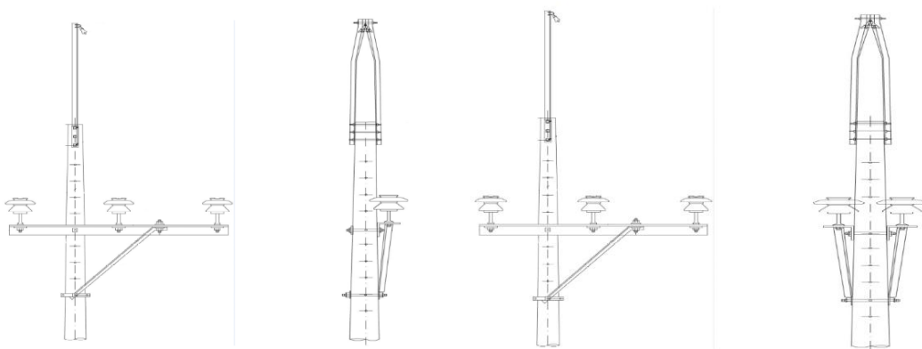
Figura 2.138 Esquema tipo de estructura de paso con ángulo de deflexión 0-5 grados y de hasta 10 grados
