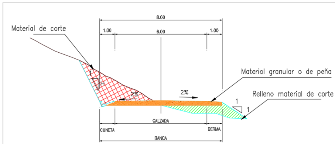
Figura 2-44. Sección transversal de vía a construir.
