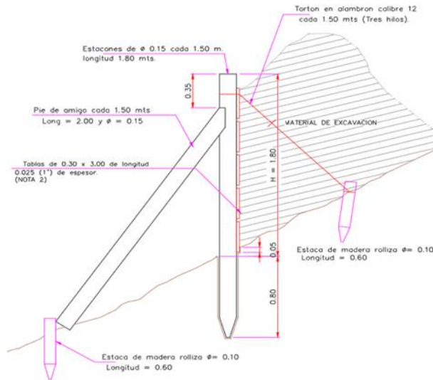
Figura 2-70 Trinchos
