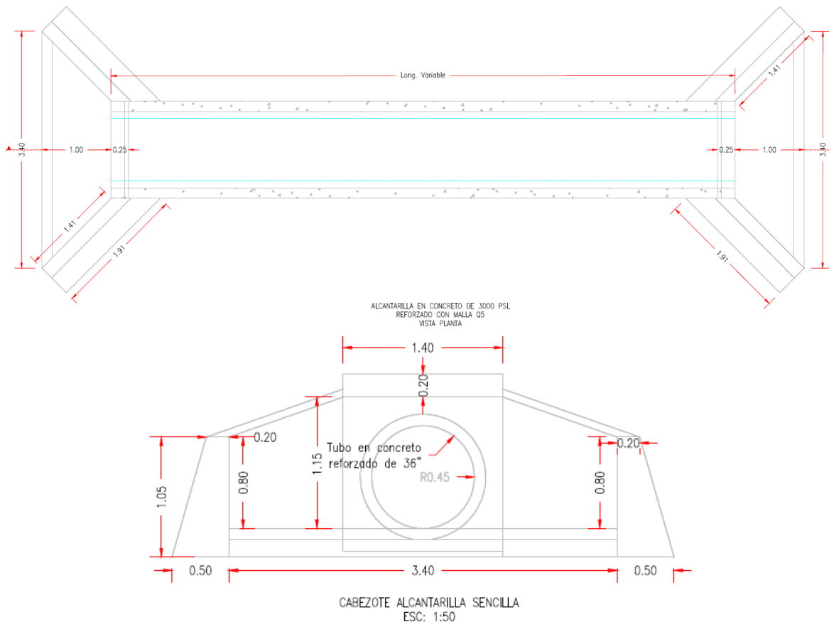
Figura 2-50 Alcantarillas
