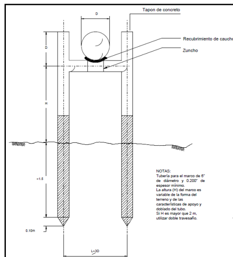
Figura 2-89 Esquema tipo Marco H
