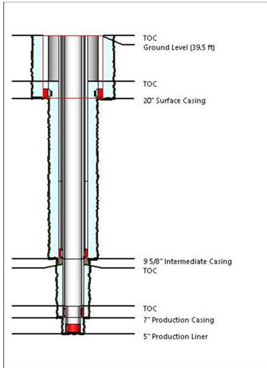
Figura 2-74 Estado mecánico tipo de la perforación de pozo inyector y/o reinjector
