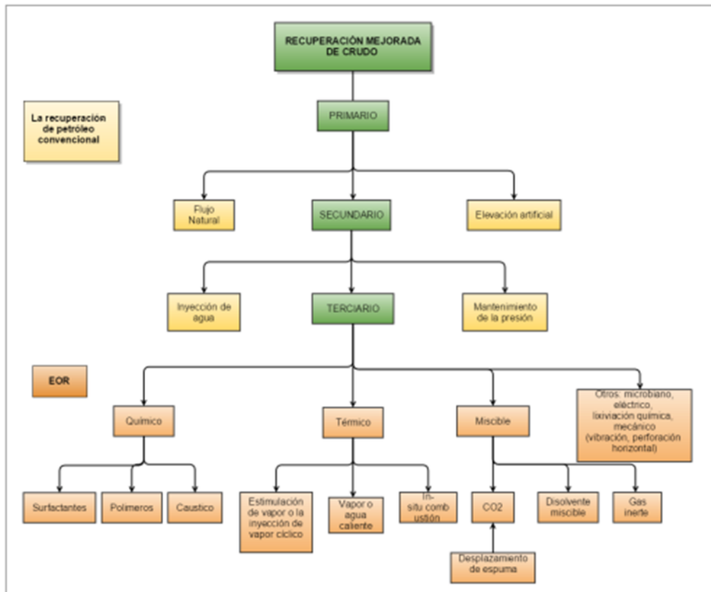
Figura 2-85 Etapas de la recuperación mejorada de crudo
