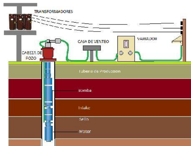
Figura 2-83 Esquema tipo del sistema de Bombeo Electrosumergible
