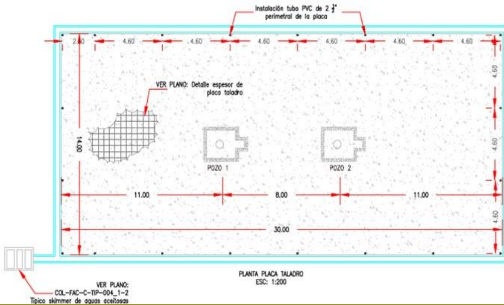
Figura 2-63 Placa de equipos
