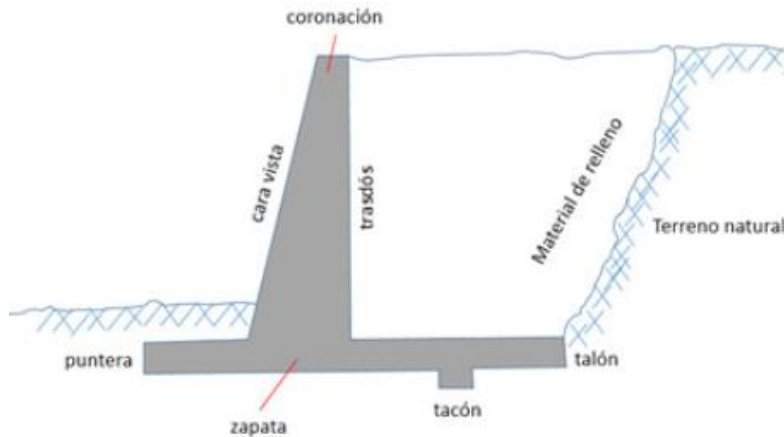
Figura 2-69 Muro de contención
